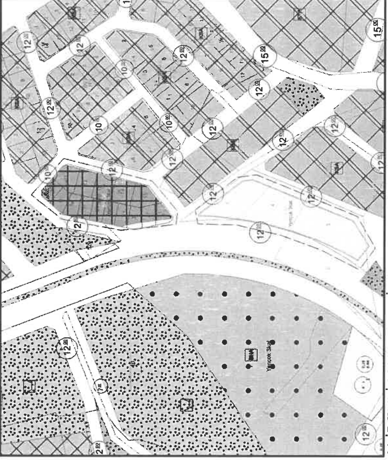
ALİBEYLİ MAHALLESİ, 899 ADA VE 196 ADA 3, 4, 5 PARSELLER ÖNERİ İMAR PLANI
