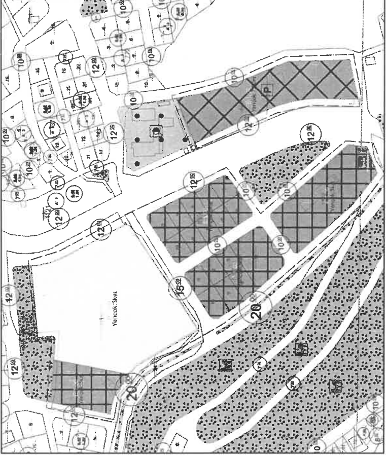
CAMİİ KEBİR MAHALLESİ, 1120, 838, 839, 1118 ADALAR VE 1039 ADA 4 PARSEL, ÖNERİ İMAR PLANI
